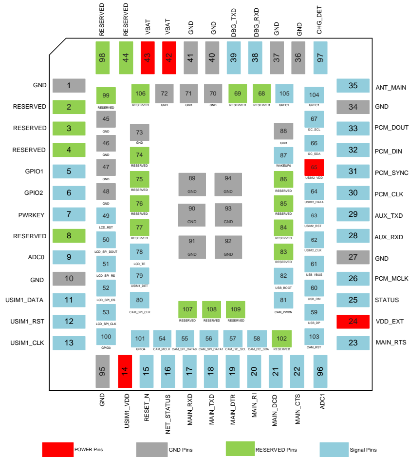
图 2: 引脚分配图
