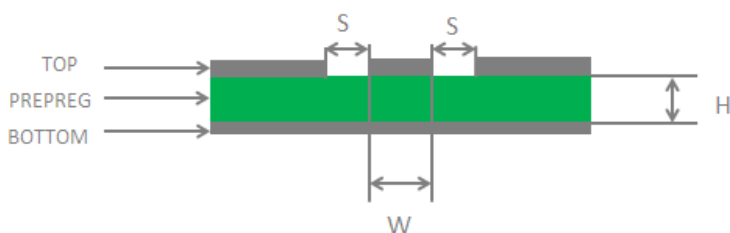
图 25: 两层 PCB 板共面波导结构
