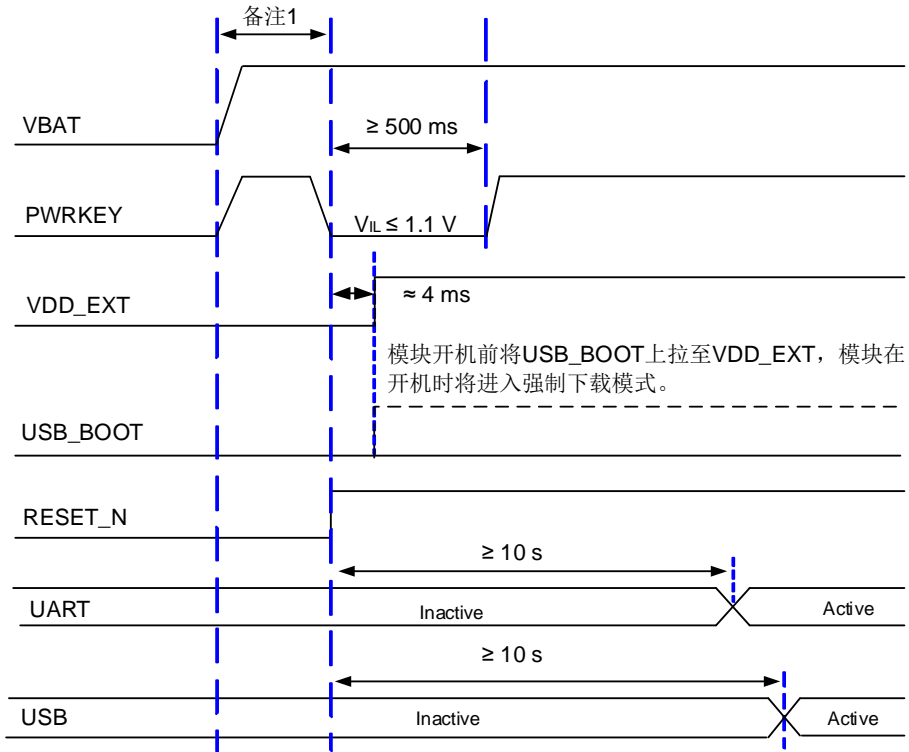
图 11: PWRKEY 开机时序图
