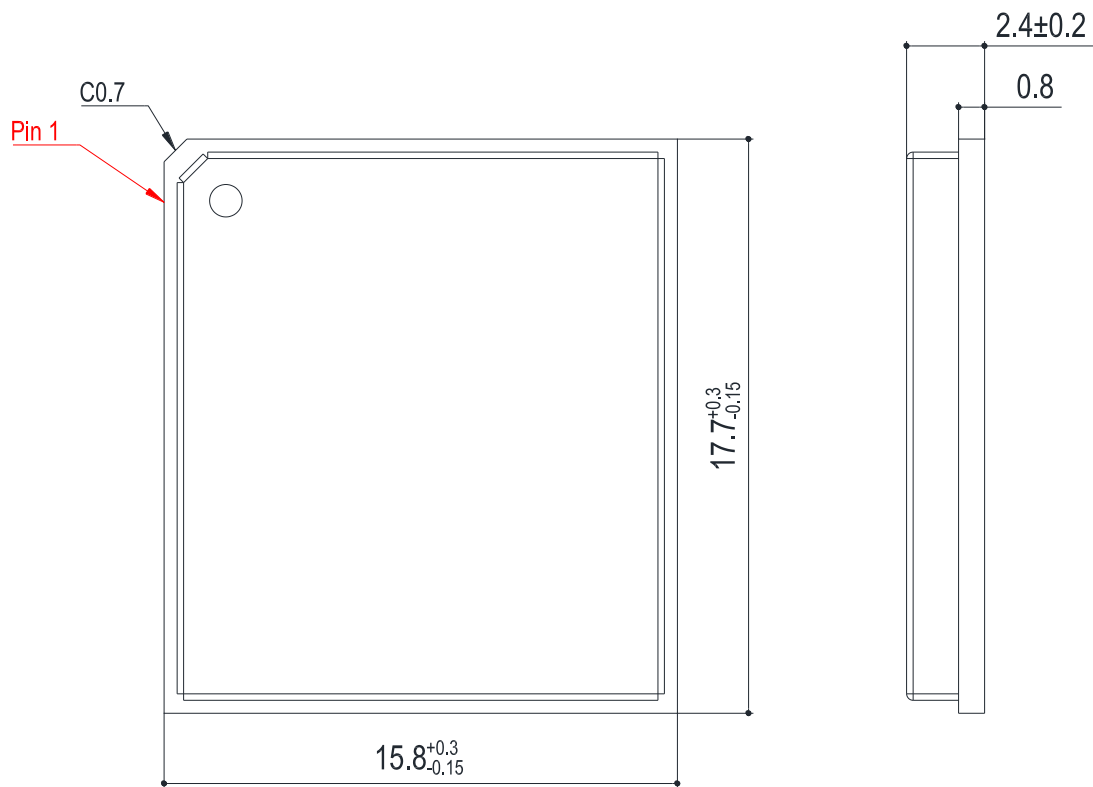
图 31：俯视及侧视尺寸图（单位：mm）
