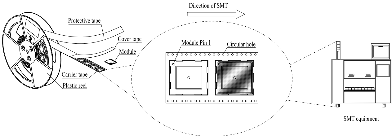
图 38: 贴片方向
