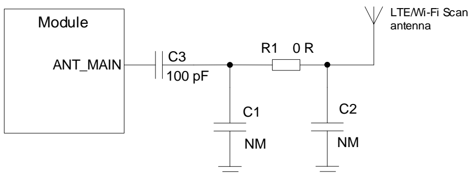
图 23: 射频参考设计图
