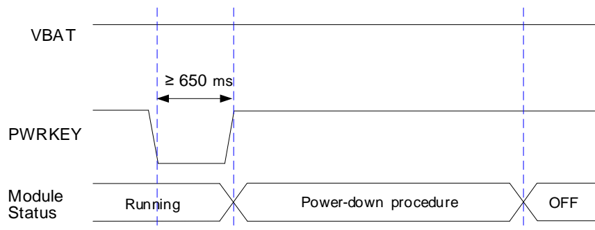
图 12: PWRKEY 关机时序图
