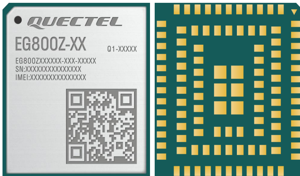
图 34: 模块俯视图与底视图
