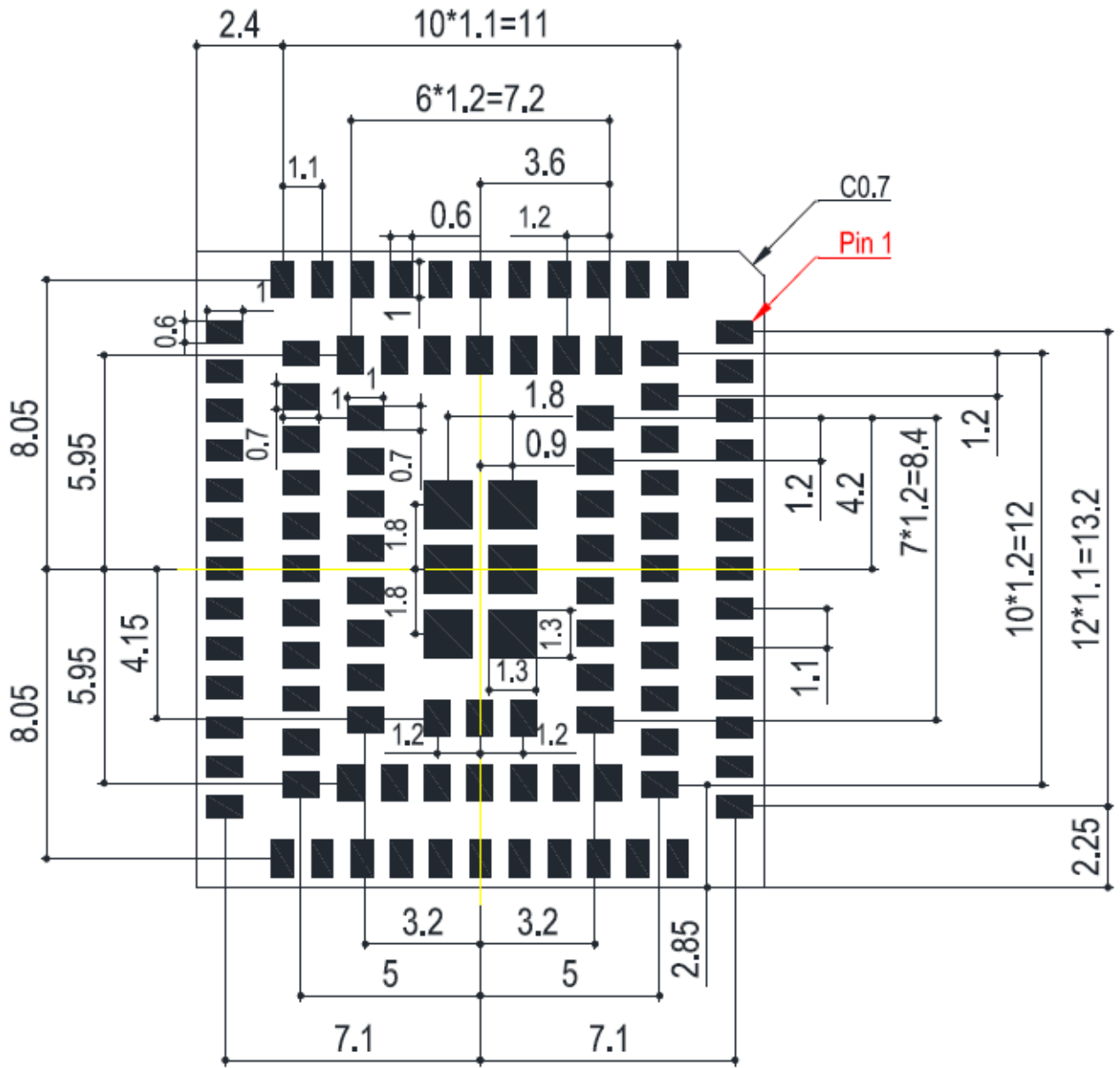
图 32: 底部尺寸图 (底视图) (单位 mm)
