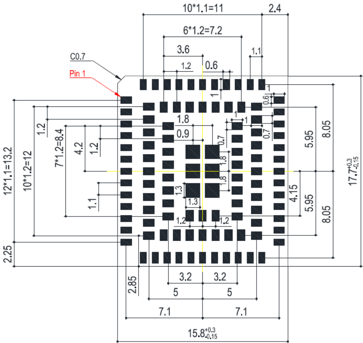
图 33: 推荐封装 (单位 mm)
