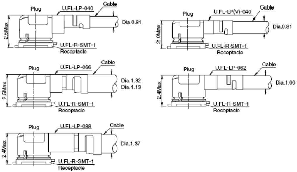
图 30: 射频连接器安装图 (单位: 毫米)
