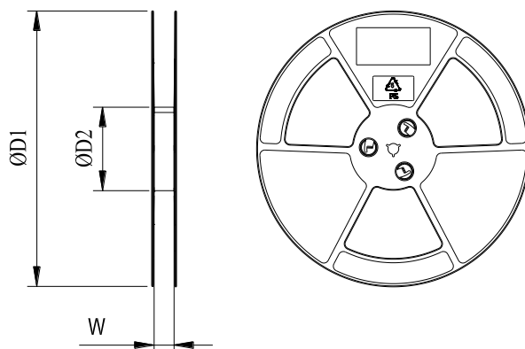
图 37: 胶盘尺寸图
