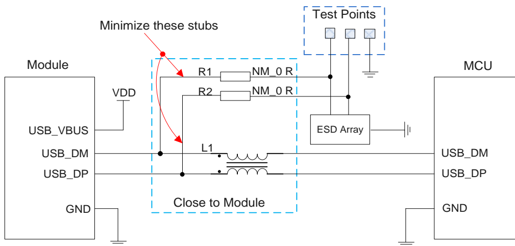
图 16: USB 接口参考电路图
