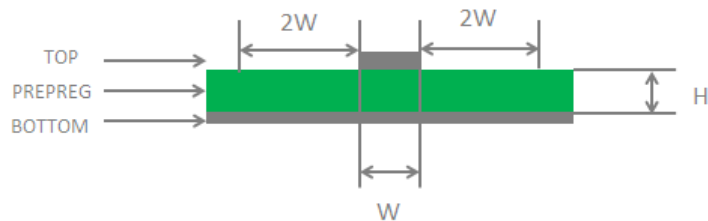
图 24: 两层 PCB 板微带线结构
