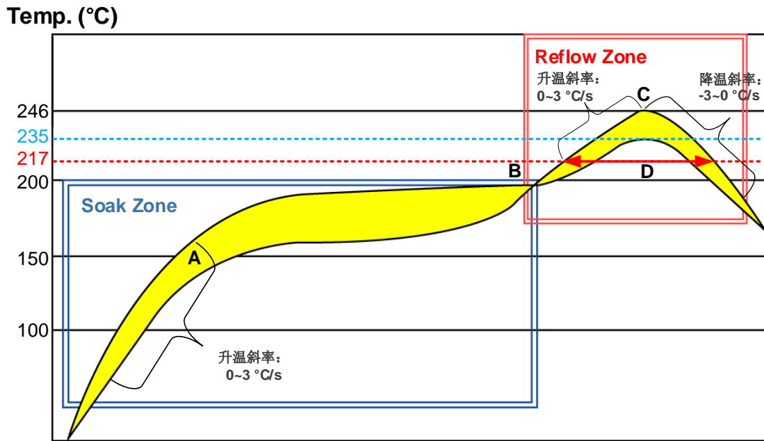
图 35：推荐的回流焊温度曲线
